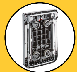
roulettes escamotables
